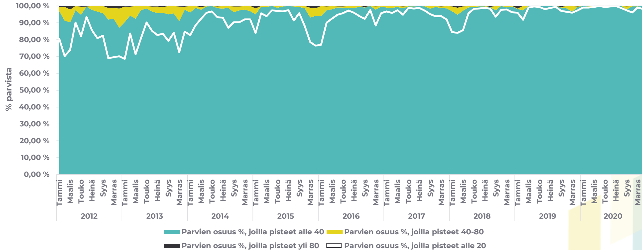
Broilereiden jalkapohjapisteet 2012-2020
